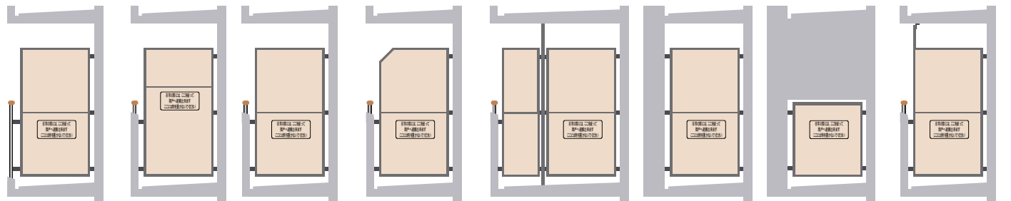
手摺り納まり (手摺支柱 + 壁)
